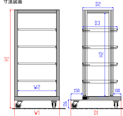
寸法図面
