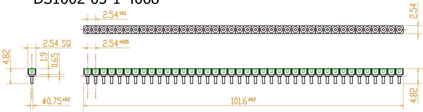
ピンヘッダー寸法図面
